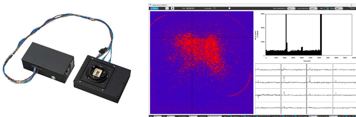
(左:MEA システムのハードウェア、右:計測アプリケーションの UI イメージ)
